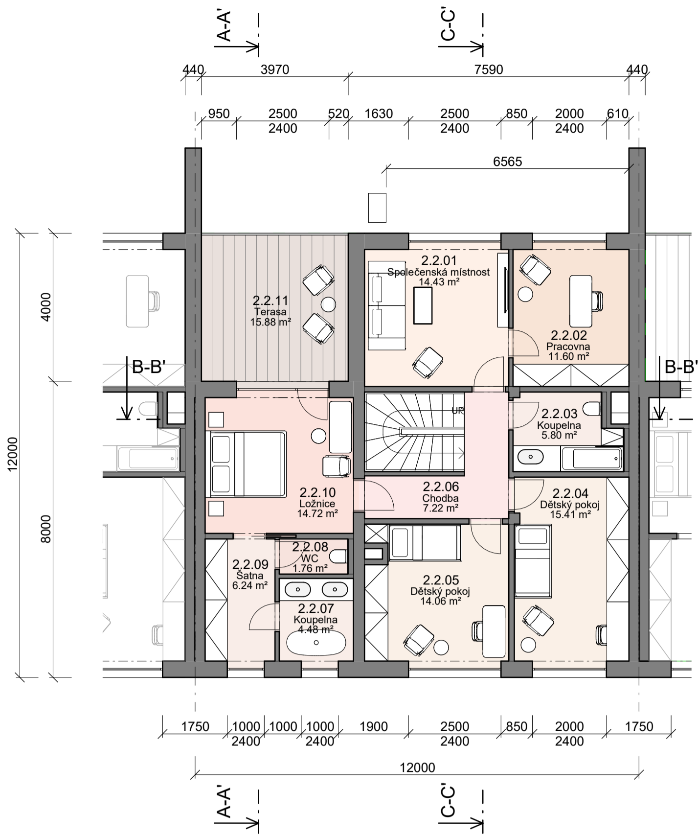
PŮDORYS 2NP
